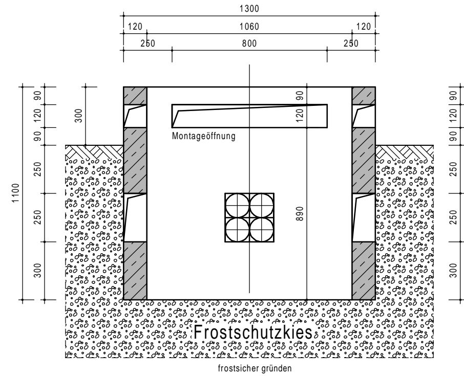
Schnitt B-B M 1:20
