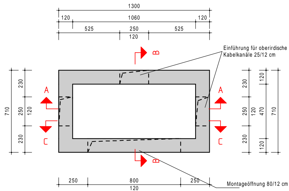
Grundriß M 1:20
