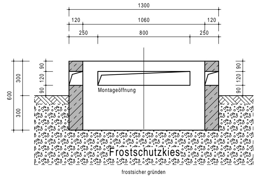
Schnitt C-C M 1:20
