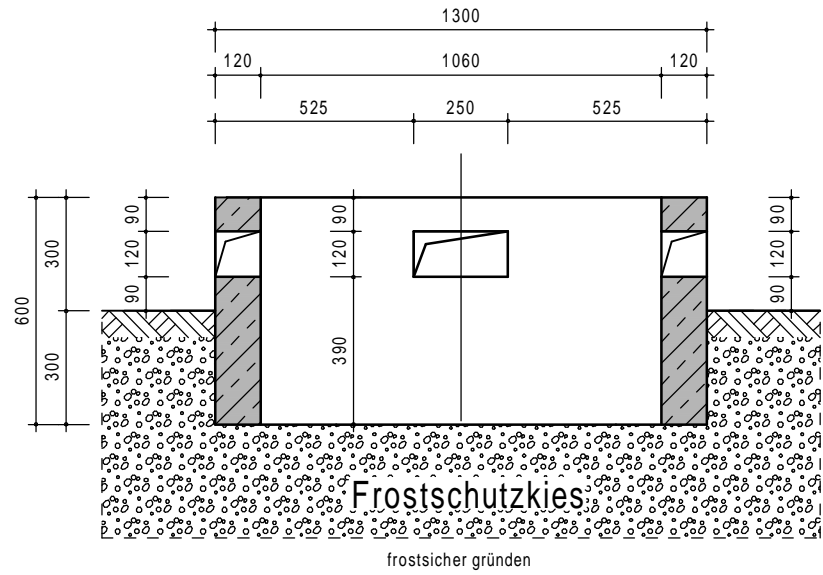
Schnitt A-A M 1:20
