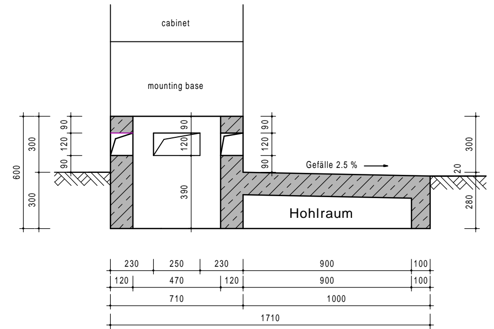
Schnitt B-B M 1:20
