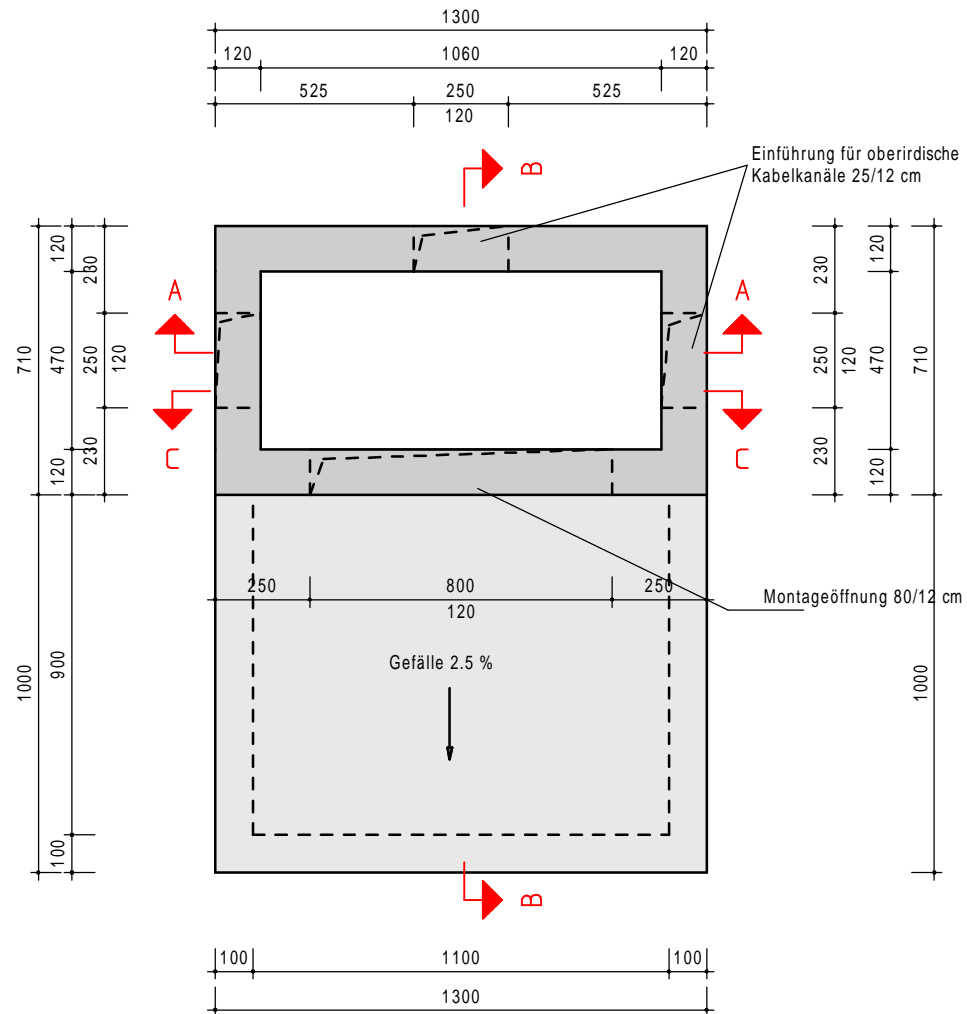
Grundriß M 1:20
